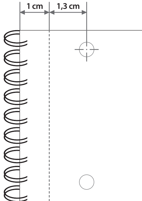
Fortrykt indvendig del med perforation (udsnit)
